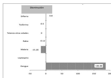
Gráfico No. 1 Reporte de enfermedades seleccionadas de notificación obligatoria, República Dominicana. Comparación de 4 semanas previas con datos históricos, últimos cinco años, 14 de agosto 2010
